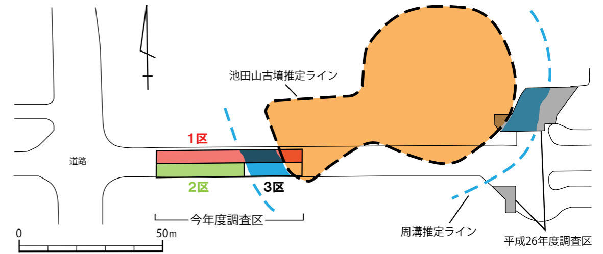
池田山古墳・塚口山廻遺跡調査区配置図
